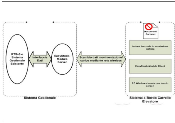
Schema funzionale di EasyStock
